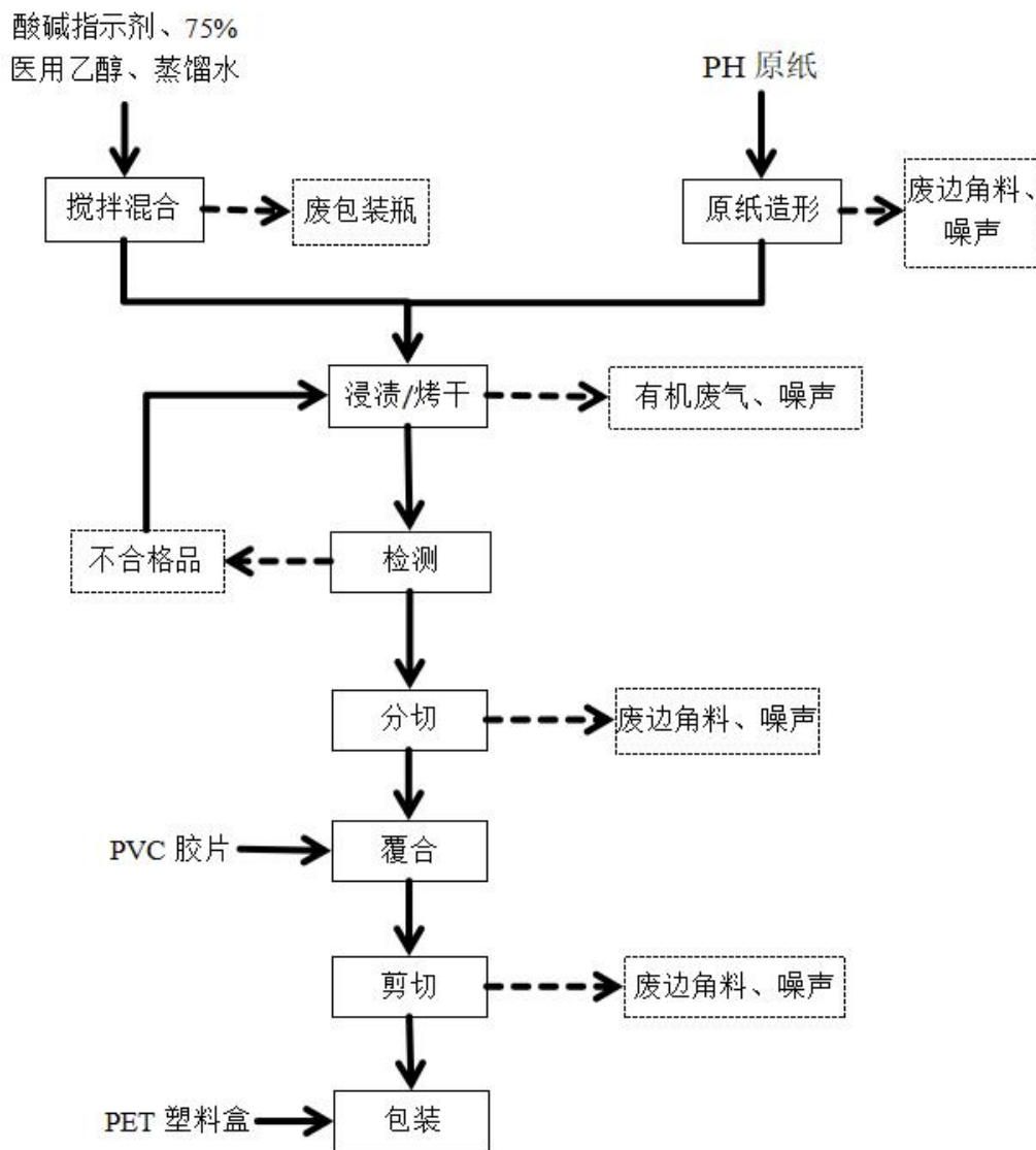
图 2 项目生产工艺流程图
