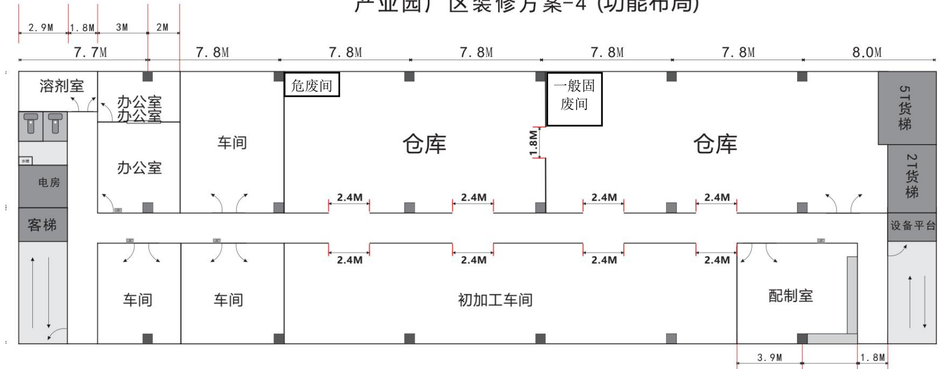
附图 4 项目车间平面布置图
